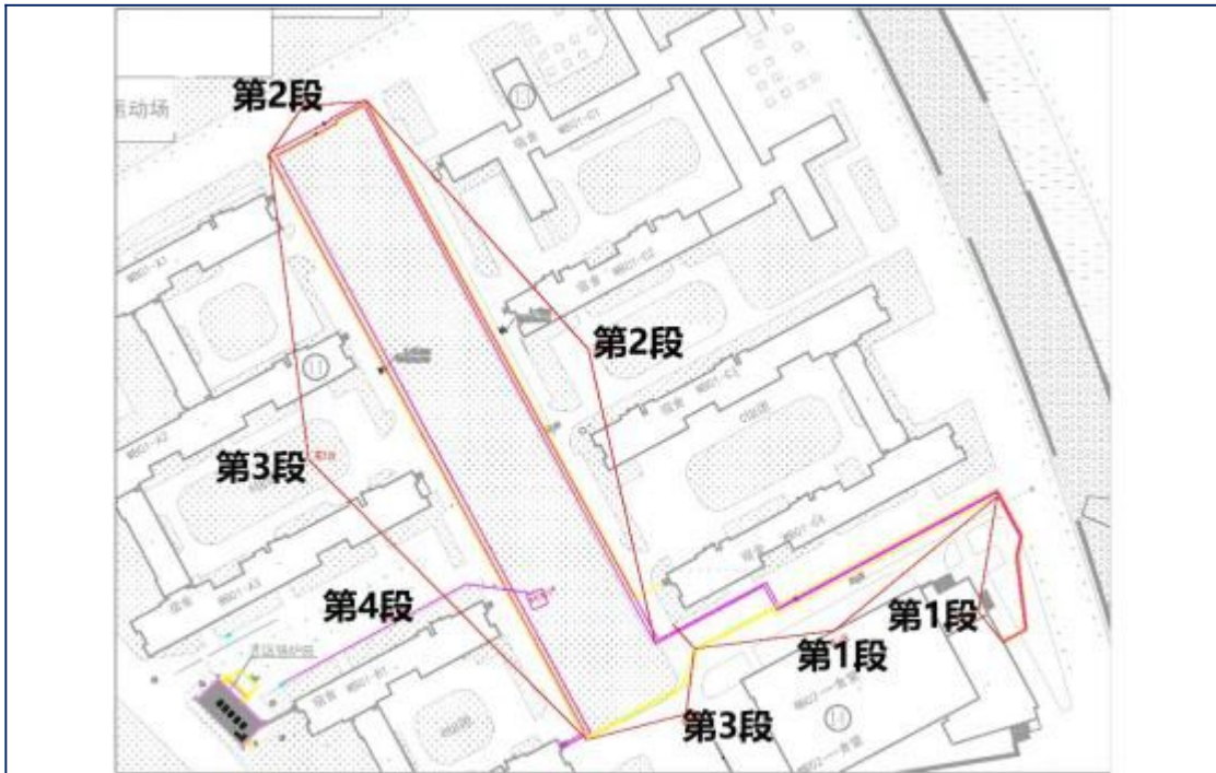
一食堂换热站至学生公寓室外管线分段施工计划图
